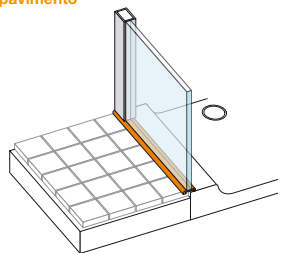
Piatto incassato filo pavimento
